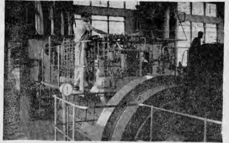
Nueva Unidad Diesel Eléctrica, con capacidad de 500 KW, que está entrando en operación en la ciudad de Puntarenas. La capacidad de las seis plantas instaladas en el Pacífico se eleva a 4008 KW.
